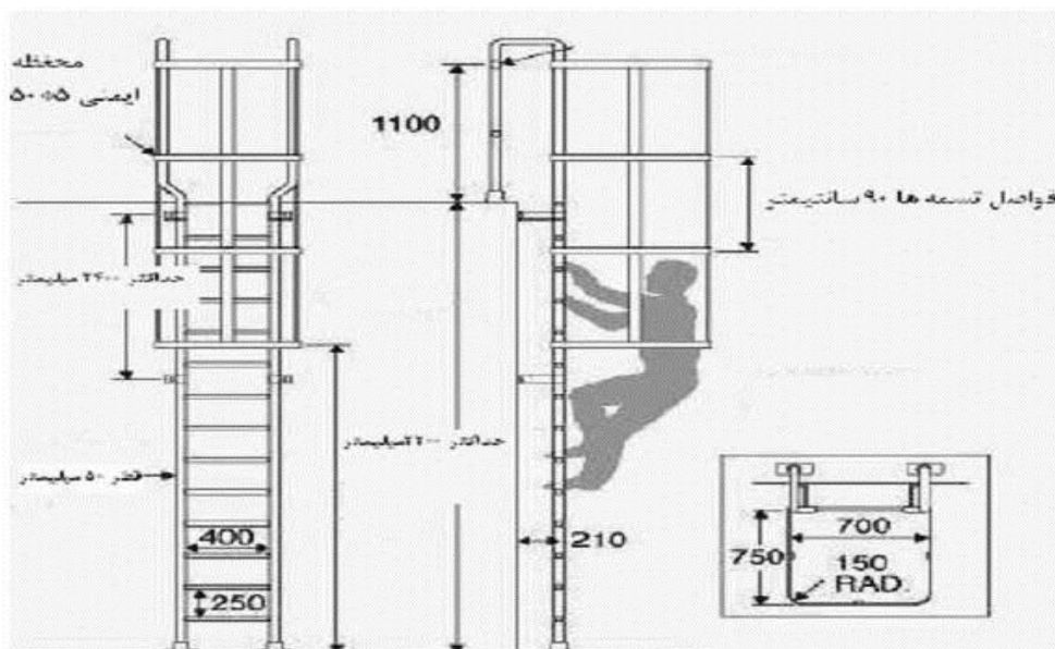
شکل ۱۷- تردد بان ثابت با محفظه حلقوی
