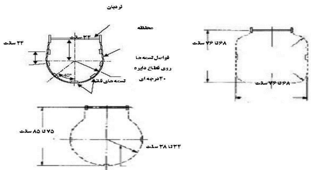
شکل ۲۱ - مختصه نود جان کابینت
